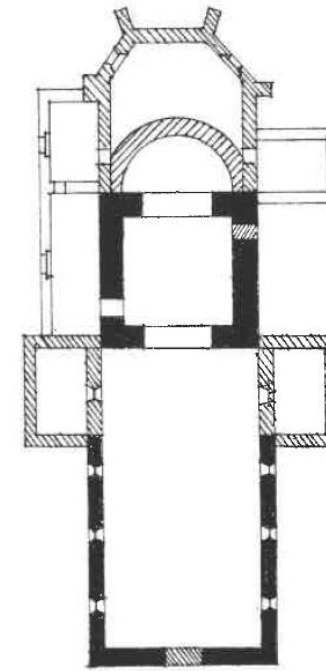
Grondplan van de kerk vóór 1847
